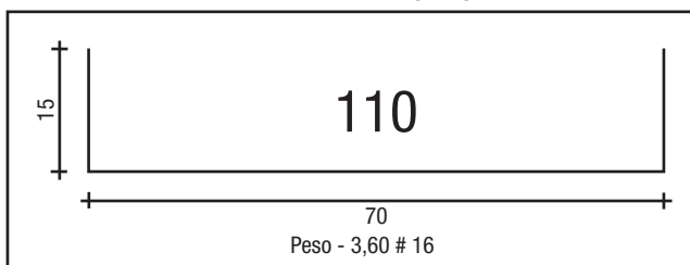
LATERAL DE 70 # 16
