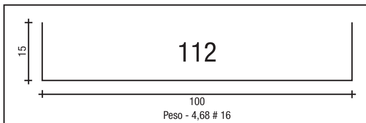
LATERAL DE 100 # 16
