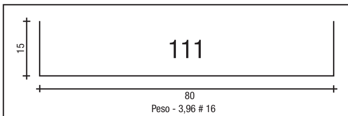
LATERAL DE 80 # 16
