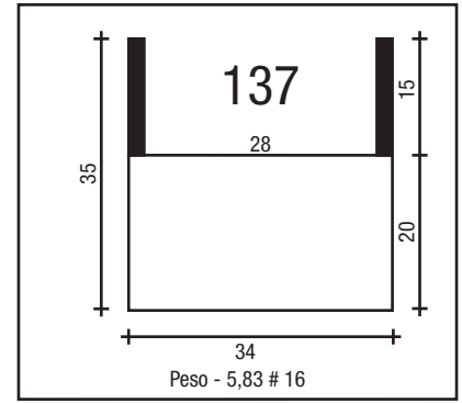
BATENTE FECH. P/ PORTA COR. 25 # 16
