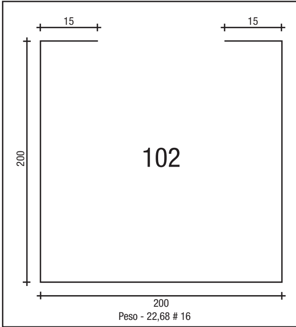
CAIXA ABERTA DE 200 # 16
