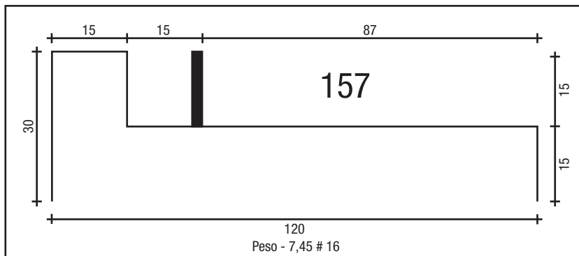
TRILHO VITRAUX 120 # 16
