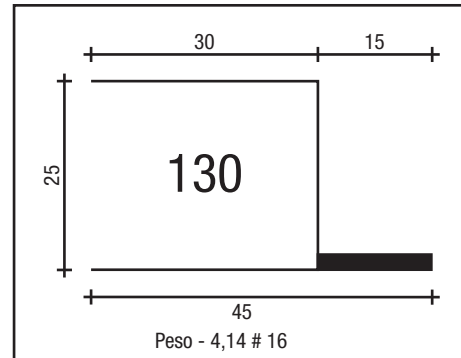
CAD. ABERTA 30 X 25 # 16
