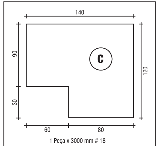
TRAVESSÃO
