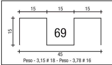
TRILHO M 45
