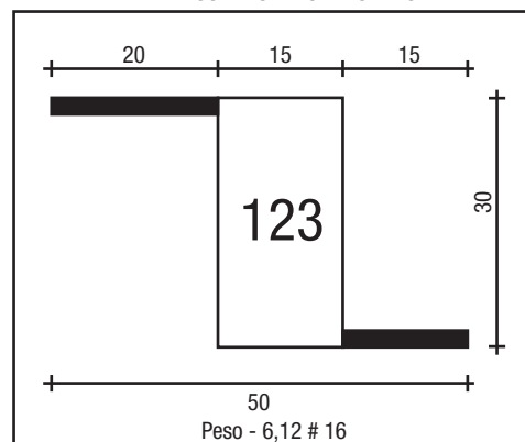
Z MAX 30 X 15 X 20 X 15 # 16
