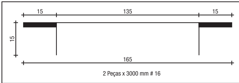
TAMPA DA COLUNA LATERAL
