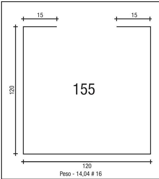
CAIXA ABERTA DE 120 # 16
