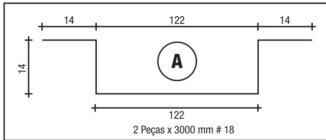
TAMPA DA COLUNA LATERAL
