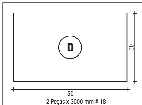
TRILHO
