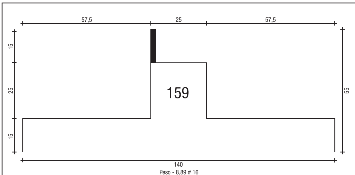
BATENTE 140 # 16
