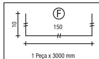
TAMPA DO TRAVESSÃO
