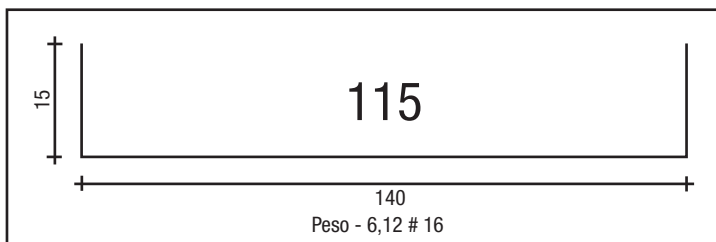
LATERAL DE 140 # 16
