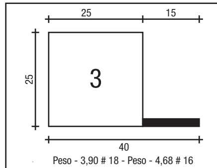
CADEIRINHA 25 X 25
