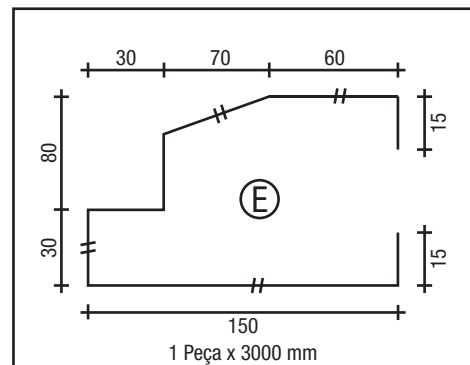
TRAVESSÃO
