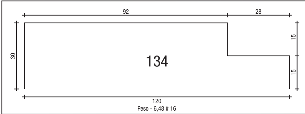
BATENTE 120 X 25 # 16
