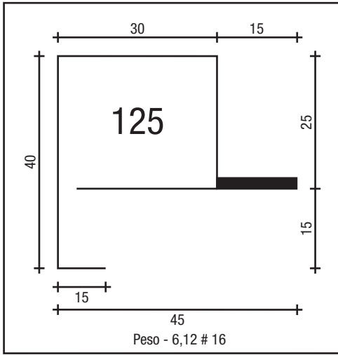
CAD. TRAVA P/ BAIXO 30 X 25 # 16
