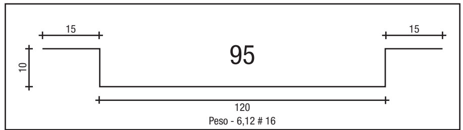
TAMPA DE CAIXA DE 150 # 16
