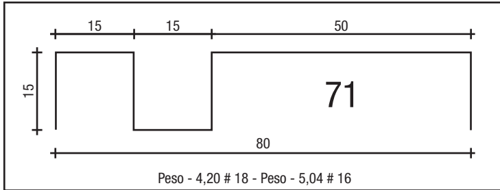
TRILHO M 80
