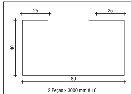
TRILHO
