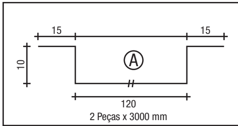
TAMPA DA COLUNA LATERAL
