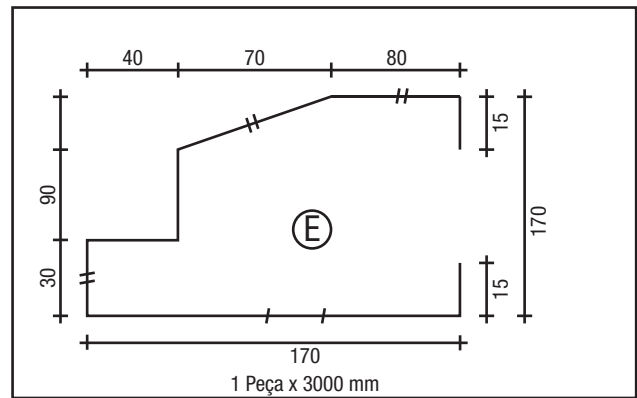
TRAVESSÃO
