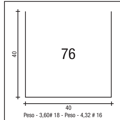
TRILHO U 40 X 40
