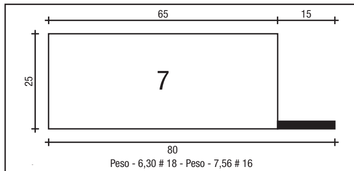
CADEIRINHA 65 X 25
