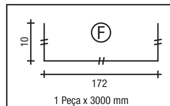
TAMPA DO TRAVESSÃO
