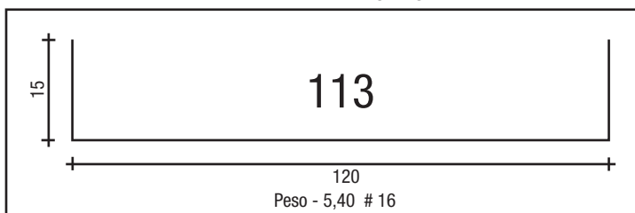
LATERAL DE 120 # 16
