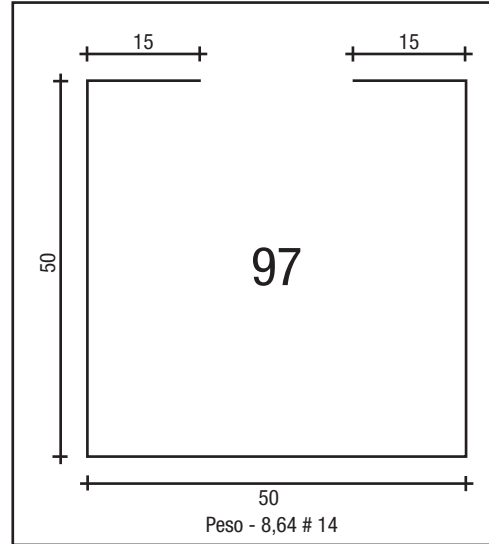
TRILHO PORTÃO ELEVAÇÃO 50 X 50 # 14
