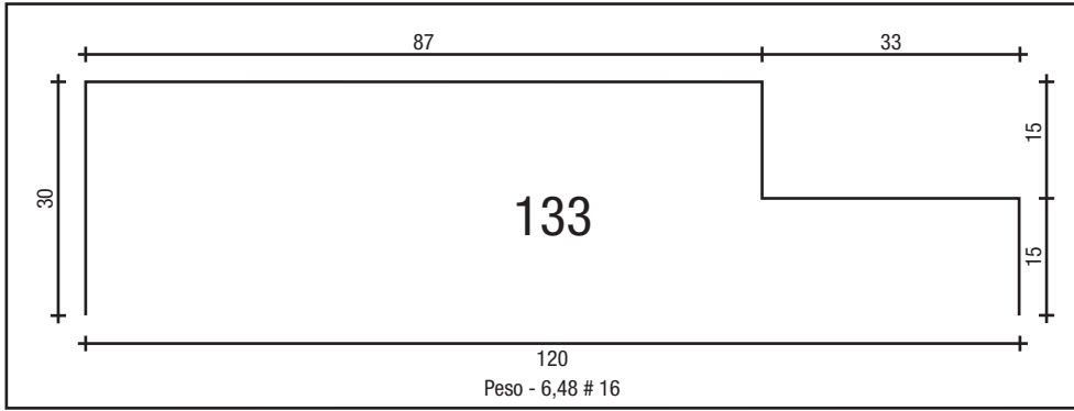
BATENTE 120 X 30 # 16
