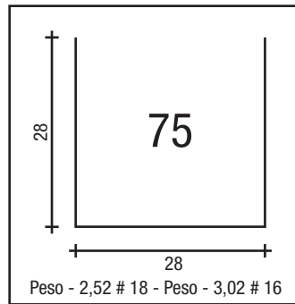
TRILHO U 28 X 28
