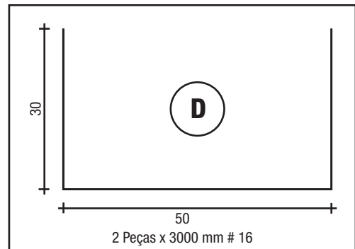
TRILHO
