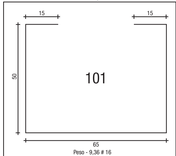
TRILHO PORTÃO ELEVAÇÃO 65 X 50 # 14
