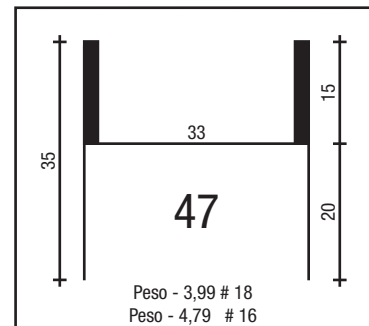
BATENTE RETO 47
