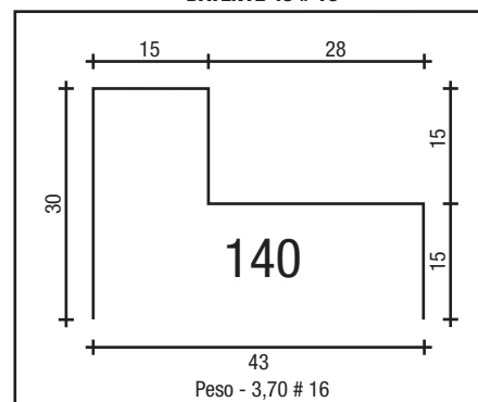
BATENTE 43 # 16
