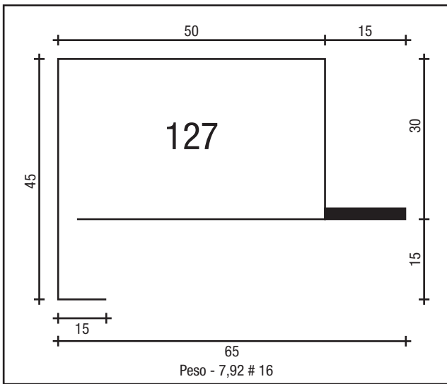
CAD. TRAVA P/ BAIXO 50 X 30 # 16
