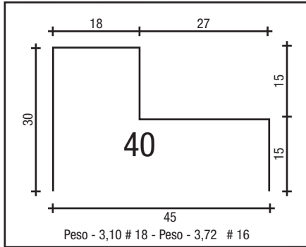
BATENTE 45
