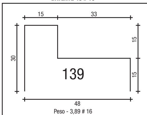
BATENTE 48 # 16
