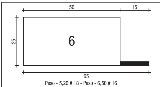
CADEIRINHA 50 X 25
