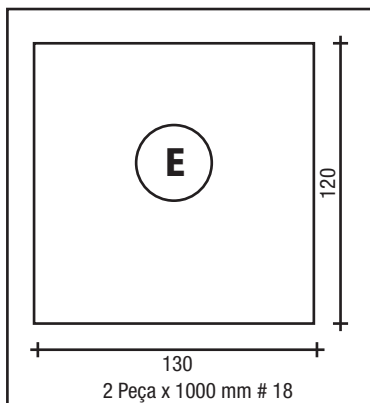
CAIXA DE PESO
