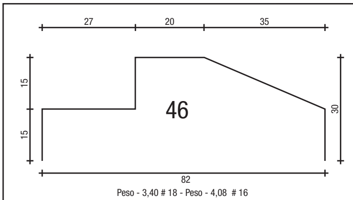
BATENTE RETO 82
