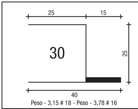
CAD. ABERTA 25 X 25
