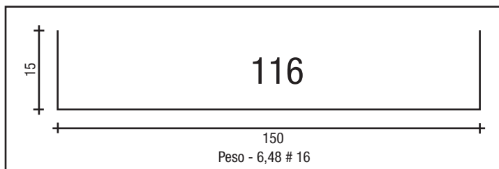
LATERAL DE 150 # 16
