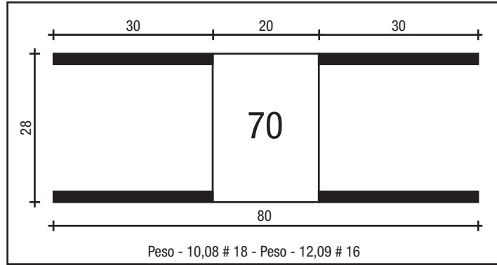
TRILHO CENTRAL
