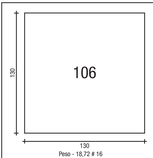
COLUNA 130 X 130 # 16
