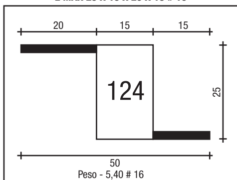
Z MAX 25 X 15 X 20 X 15 # 16
