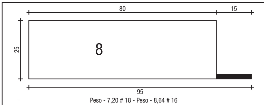
CADEIRINHA 80 X 25
