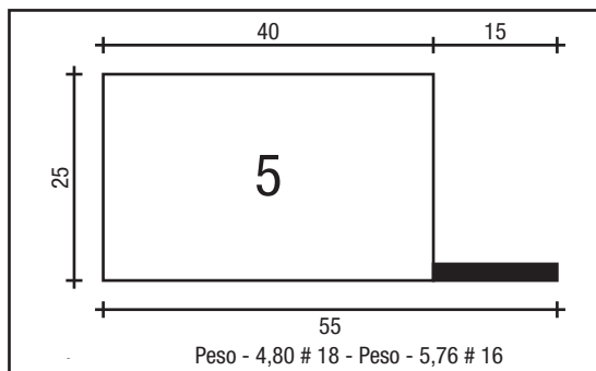
CADEIRINHA 40 X 25
