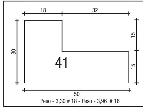
BATENTE 50
