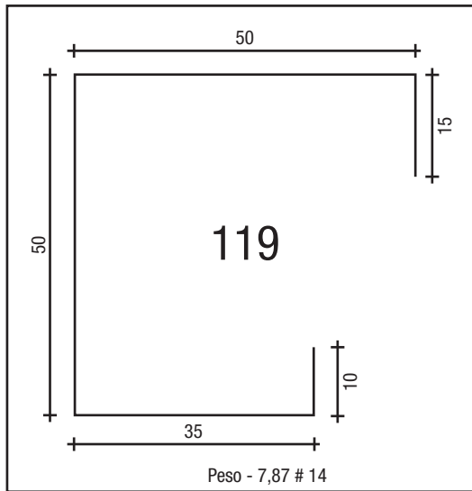
TRILHO G 50 X 50 X 35 # 14
