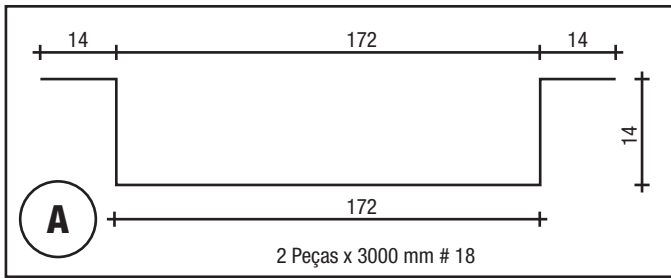
TAMPA DA COLUNA LATERAL
