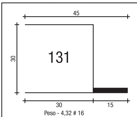
CAD. ABERTA 30 X 30 # 16
