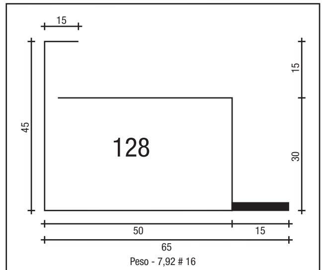
CAD. TRAVA P/ CIMA 50 X 30 # 16
