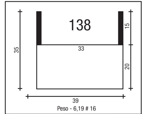
BATENTE FECH. P/ PORTA COR. 30 # 16
