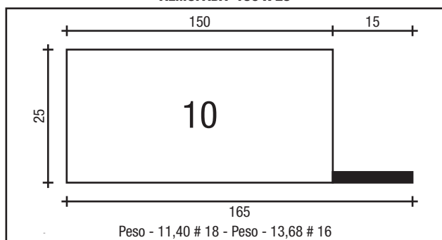
ALMOFADA 150 X 25
