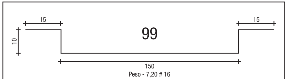
TAMPA DE CAIXA DE 180 # 16
