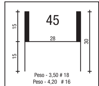
BATENTE RETO 45
