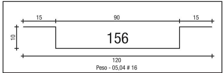
TAMPA DA CAIXA DE 120 # 16
