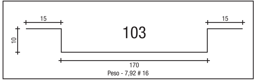
TAMPA DE CAIXA DE 200 # 16
