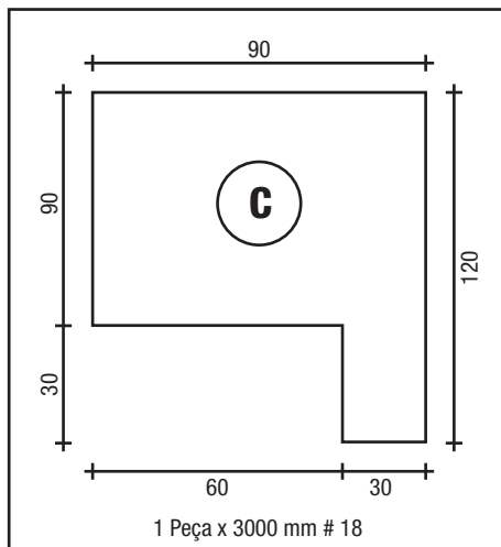
TRAVESSÃO
