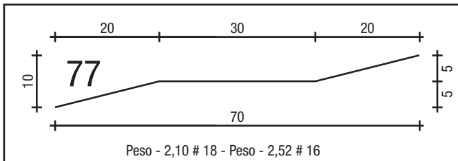
PALHETA FECHADA 10 X 15
