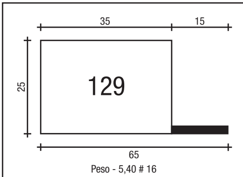
CAD. 35 X 25 # 16
