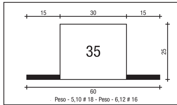
TEE 30 X 25
