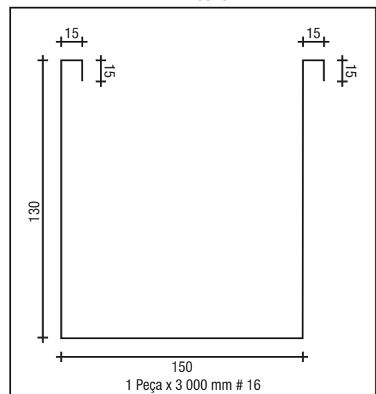
TRAVESSÃO
