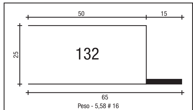
CAD. ABERTA 50 X 25 # 16
