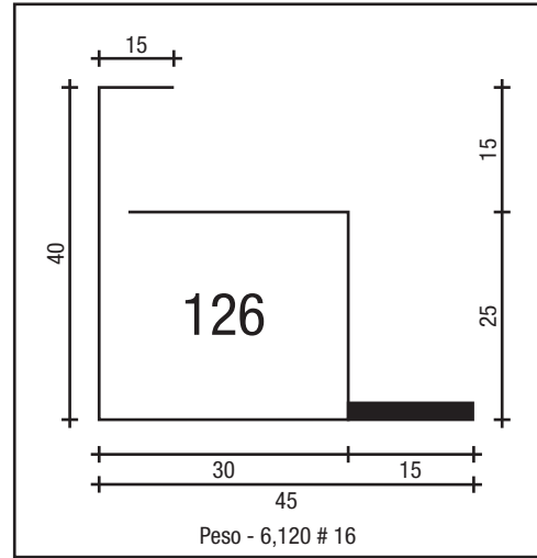
CAD. TRAVA P/ CIMA 30 X 25 # 16
