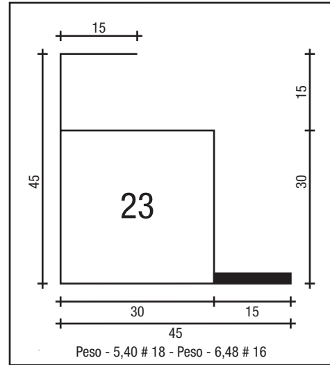
CAD. COM TRAVA 30 X 30
