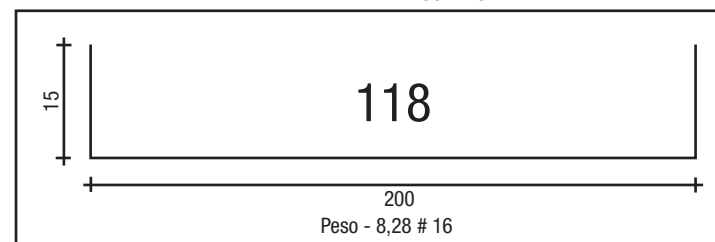
LATERAL DE 200 # 16
