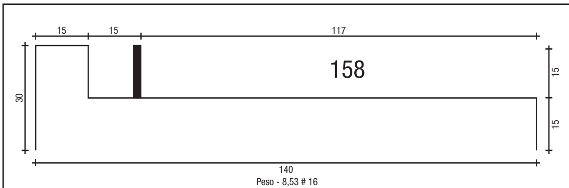
BATENTE 140 # 16
