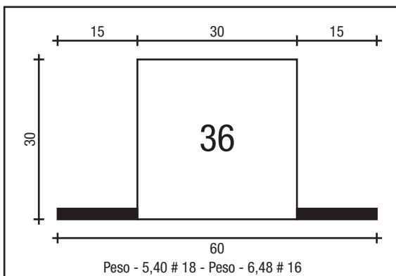
TEE 30 X 30
