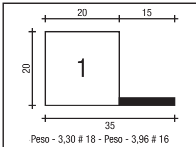
CADEIRINHA 20 X 20
