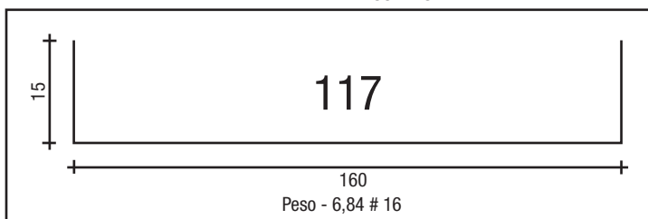
LATERAL DE 160 # 16
