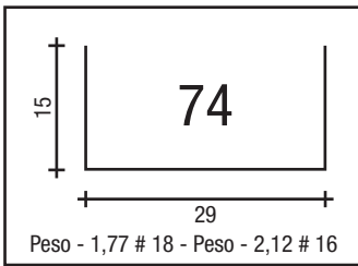
TRILHO U 15 X 29
